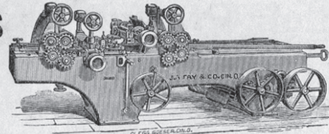
Máquina de acepillar y de machi-hembrar, Pacific No. 2½. Seis rodillos de alimentación. Cilindro doble.
