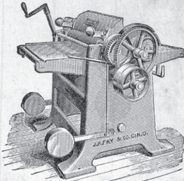
Máquina de acepillar, Centennial No. 2. 16", 20", y 24" pulgadas.
