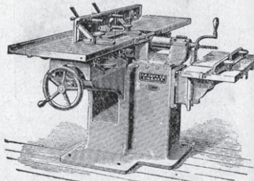
Torno "Variety" para maderas, No. 2.
