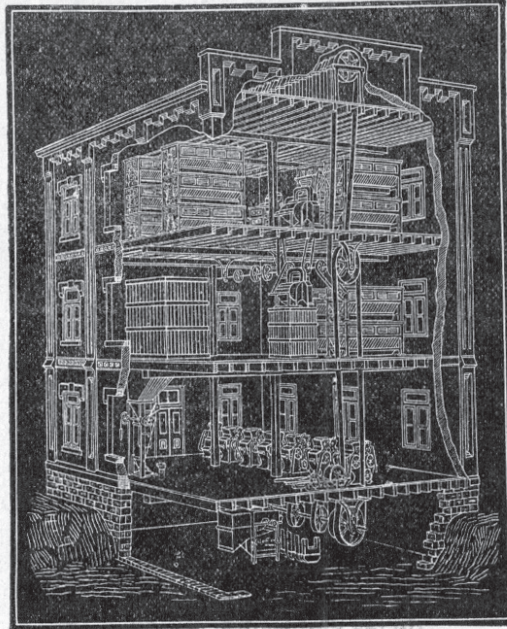
Plano de un molino completo del sistema de cilindros para harina. Pídanos la descripción de nuestros molinos modernos de cilindros.
